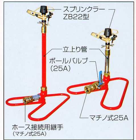
◎ 上記写真のスプリンクラーの型式・立上り管の種類・ベースの型・ホース接続用継手は、選べます。
